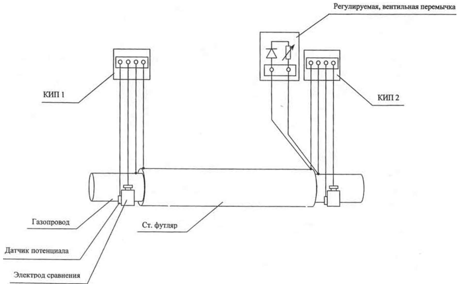
Рис.7. Схема размещения КИП при длине стального футляра более 20 м
