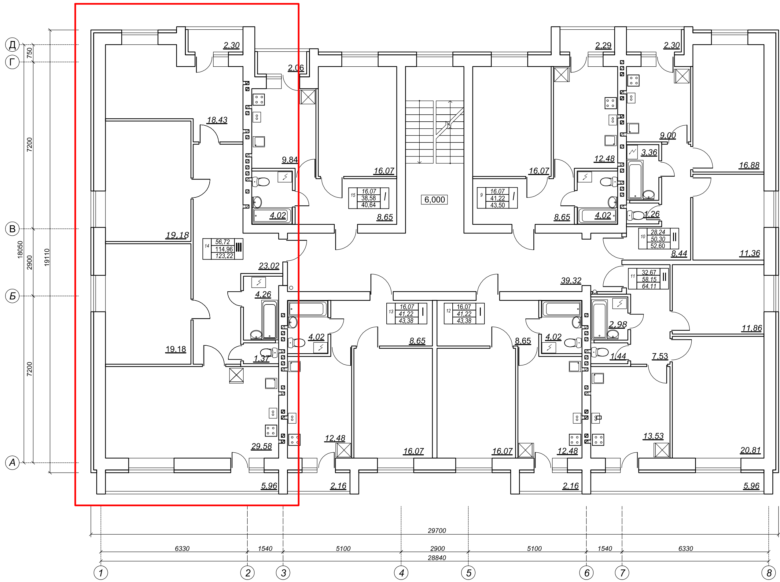
План 3-го этажа
