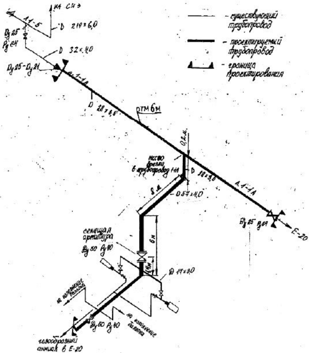
Схема трубопровода жидкого аммиака.
