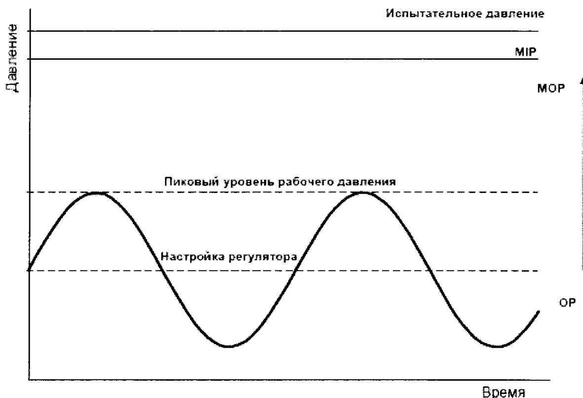
Рисунок 1 – Соотношение давлений
